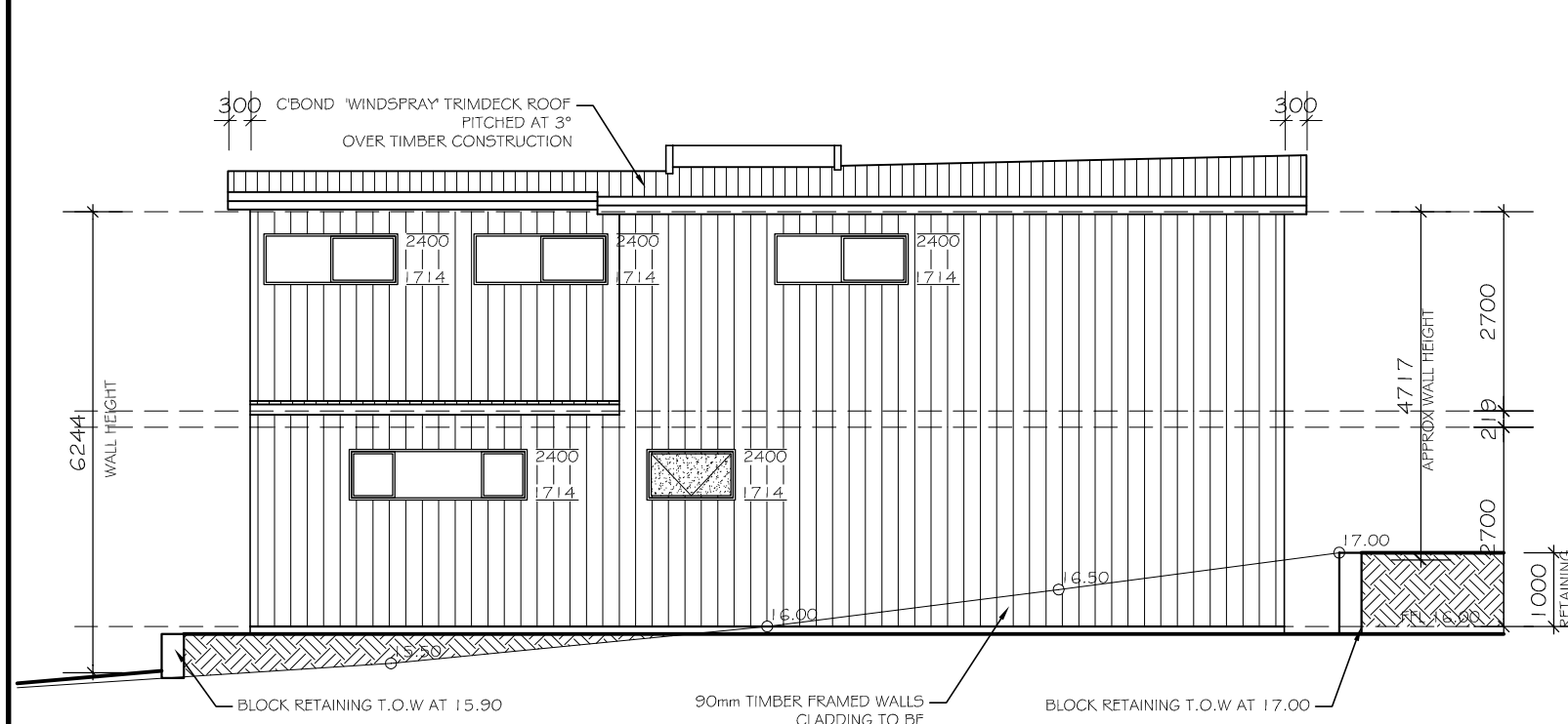
ELEVATION 3 1:100
