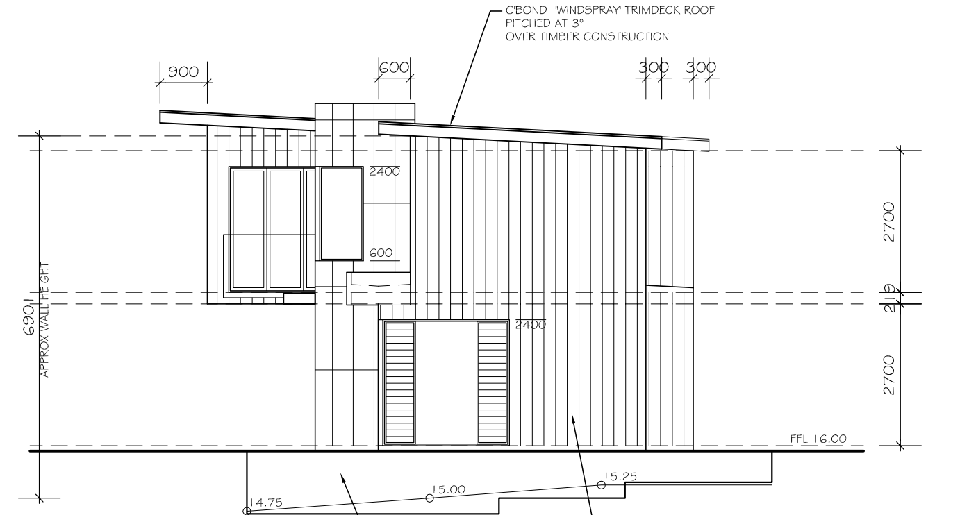
ELEVATION 4 1:100
