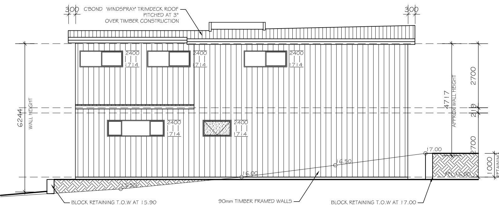
ELEVATION 3 1:100
