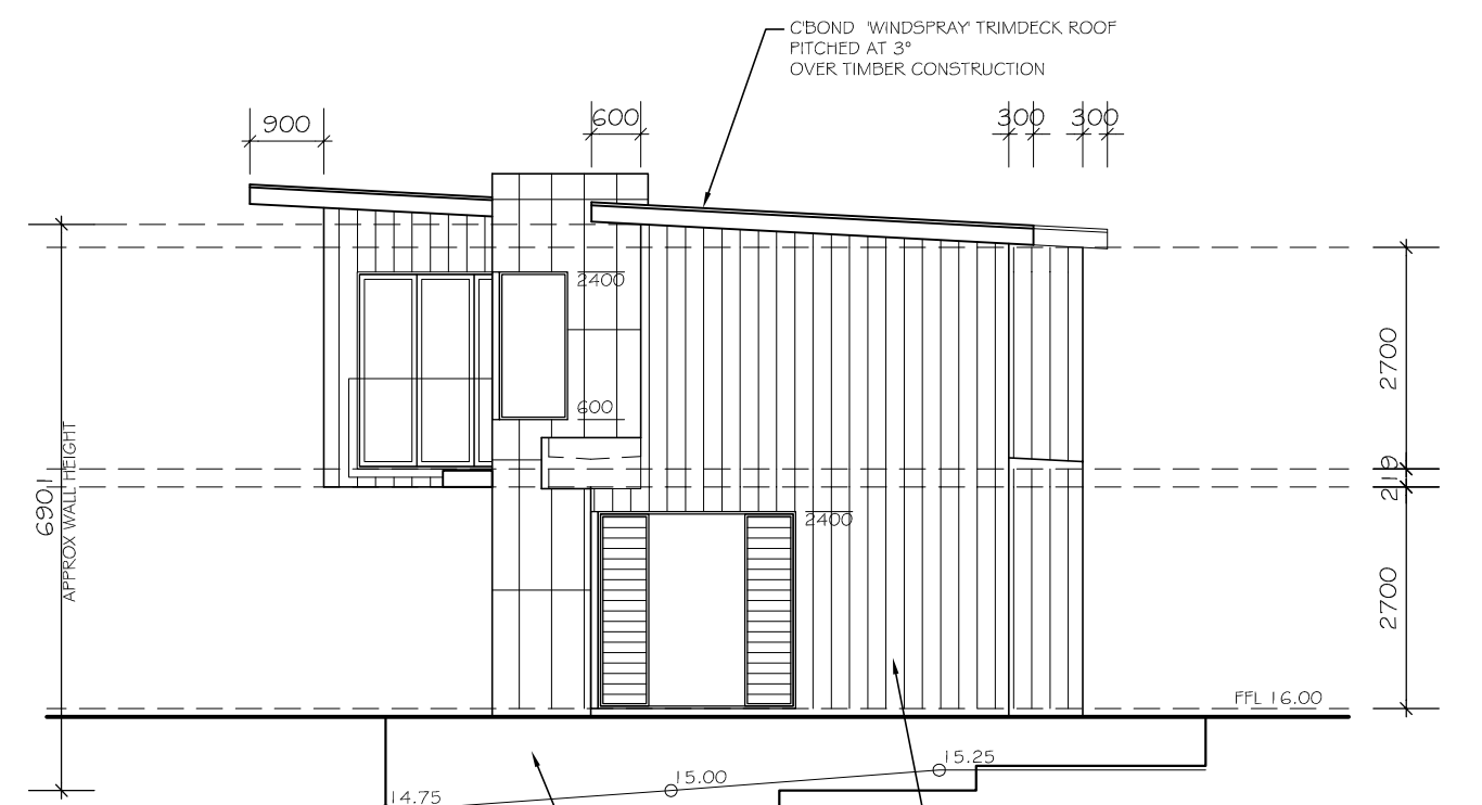
ELEVATION 4 1:100
